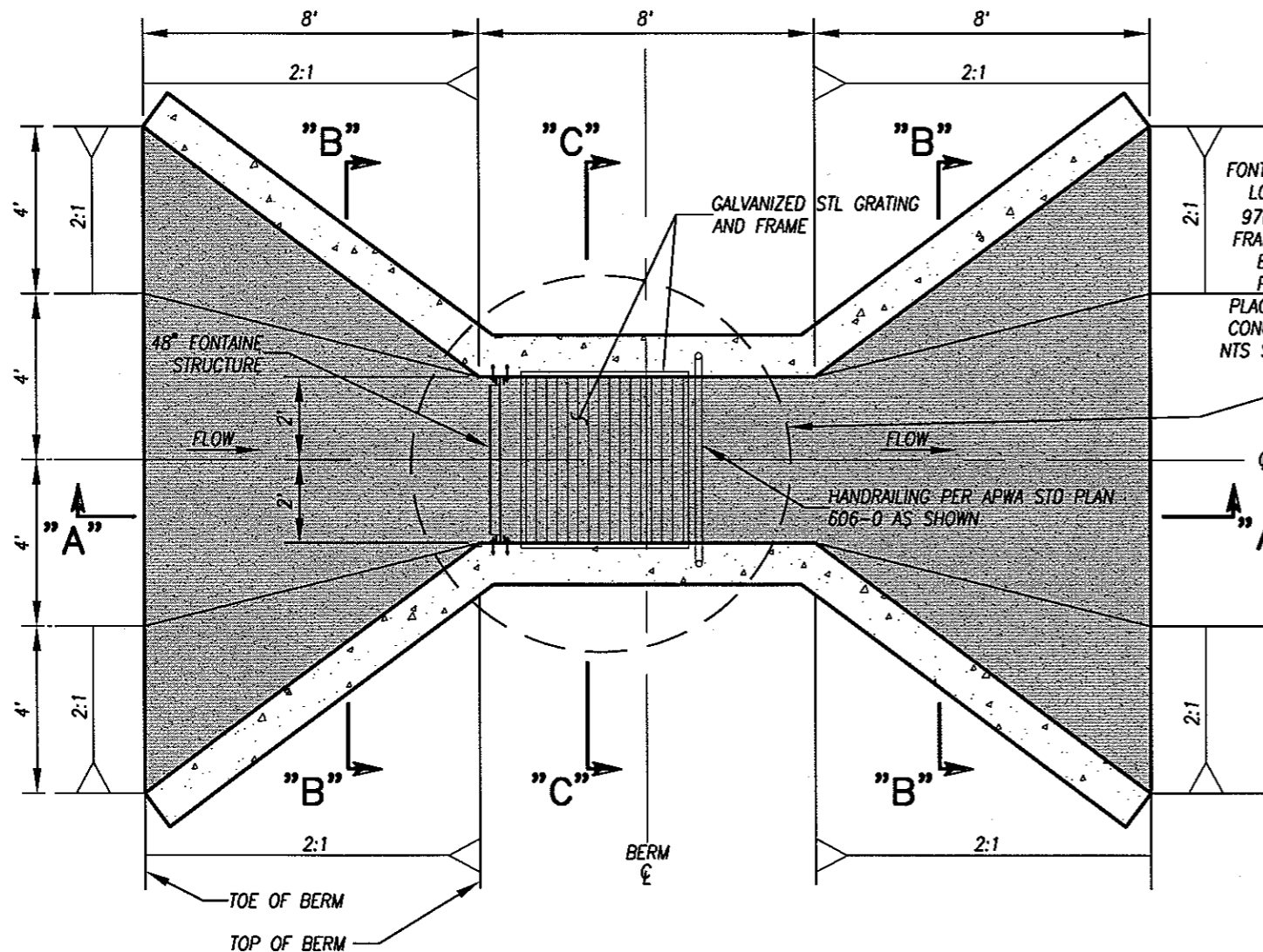
PLAN SCALE: 1" = 4'-0"
