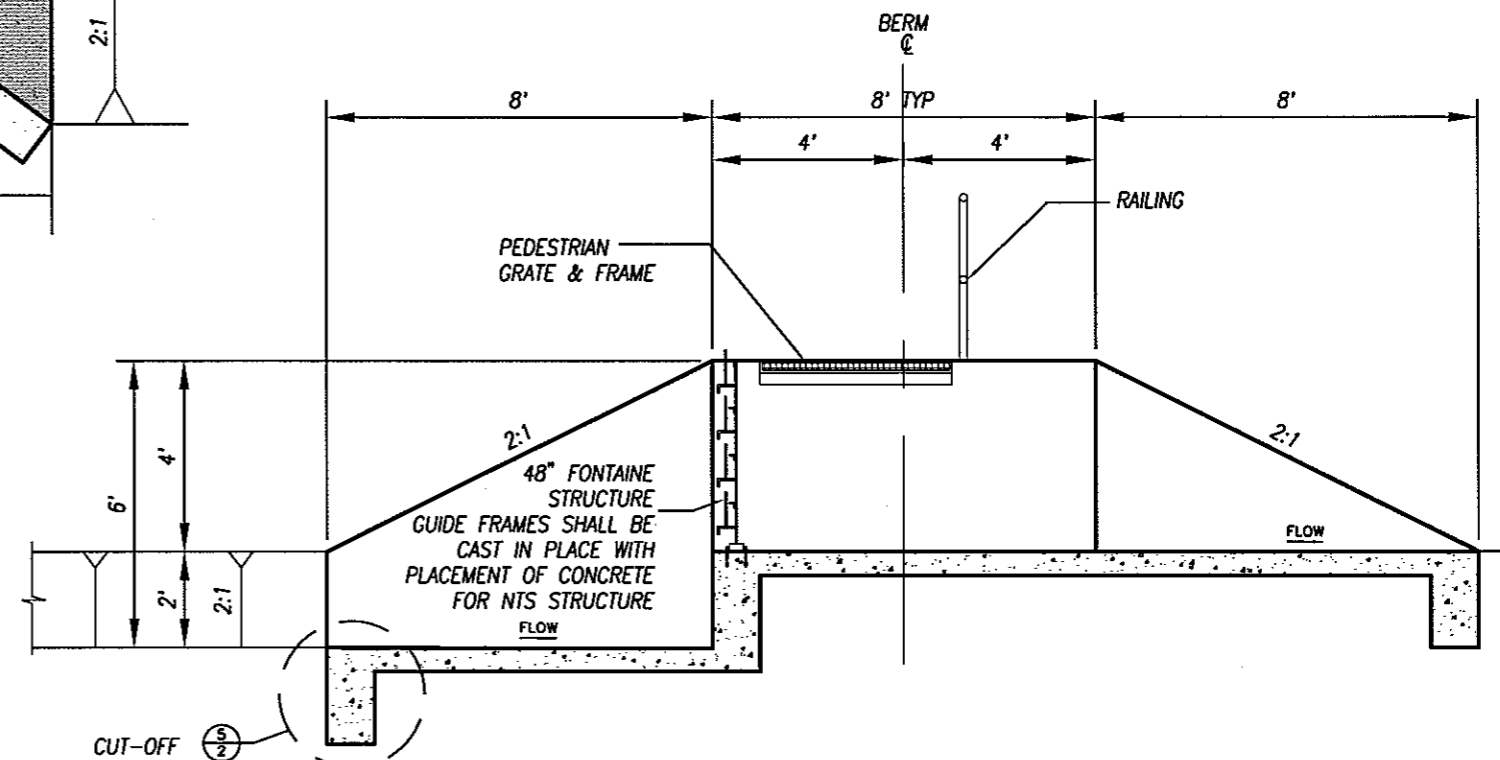
SECTION A-A SCALE: 1" = 4'-0"
