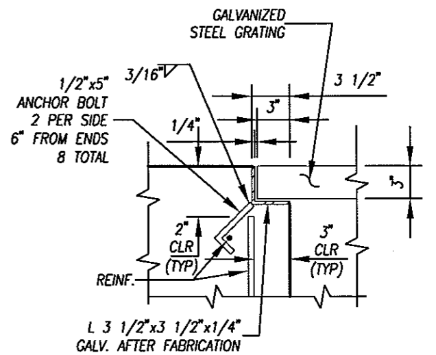
DETAIL GRATING FRAME 2 N.T.S.
